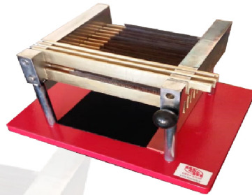
شانه اندازه گیری طول الیاف پشم
